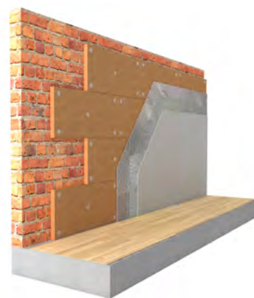
Figura 2 Esempio di una soluzione per cappotto termico interno naturale realizzato in fibra di legno Fibertherm® protect
